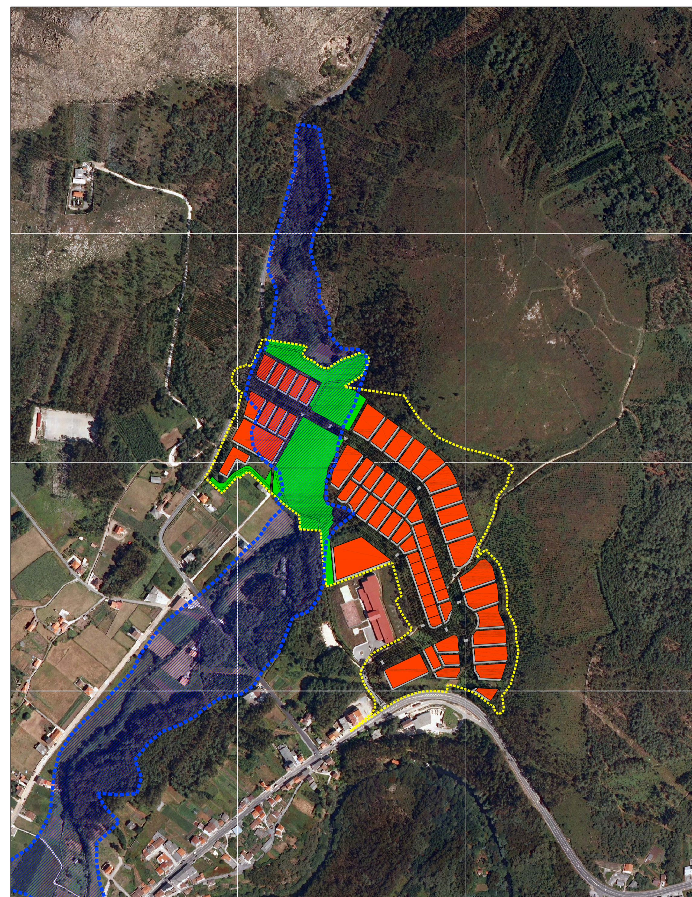
IMPLANTACIÓN PARQUE EMPRESARIAL SOBRE ORTOFOTO Escala.- 1:4.000
