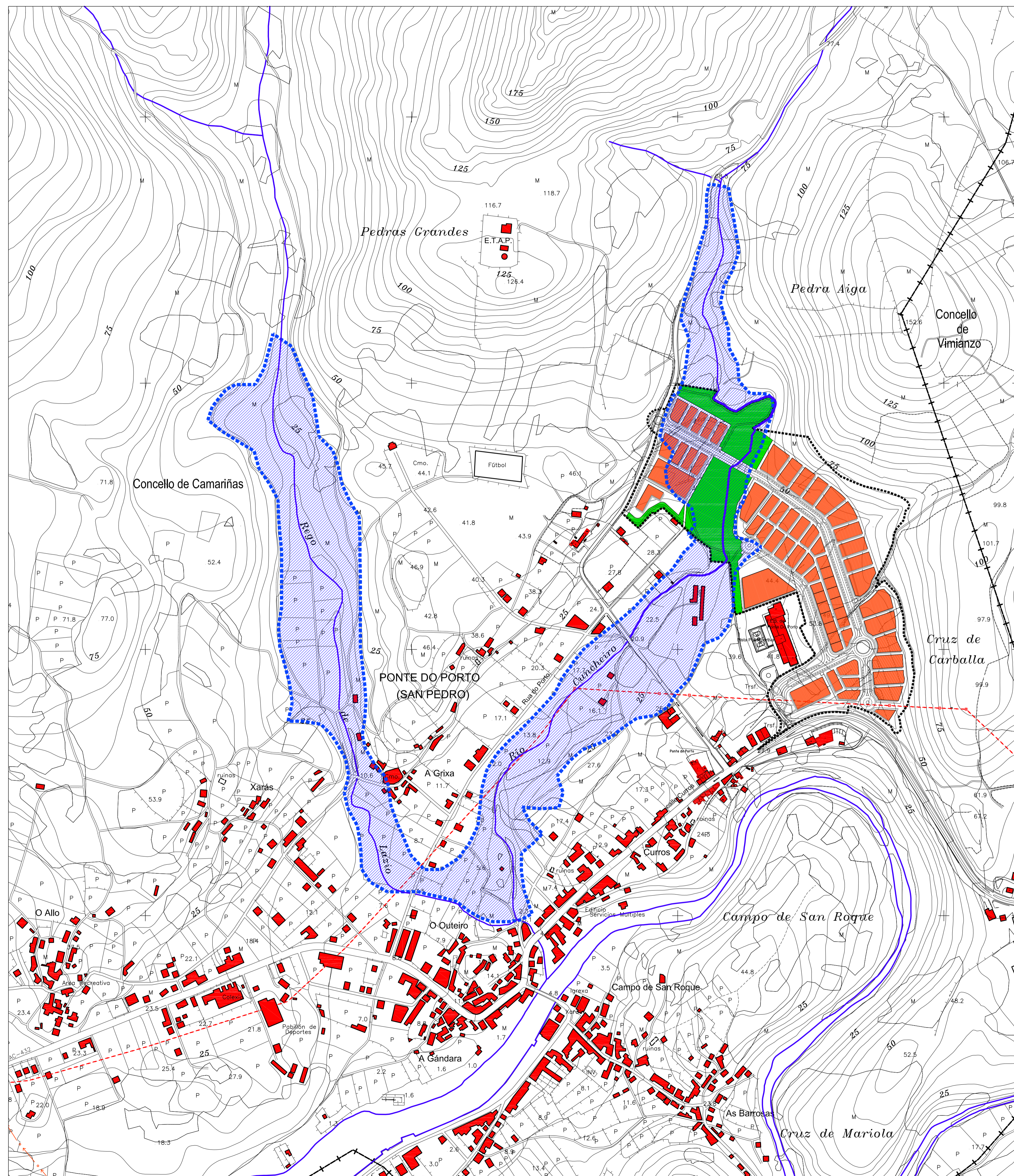
IMPLANTACIÓN PARQUE EMPRESARIAL SOBRE CARTOGRAFÍA Escala.- 1:4.000
